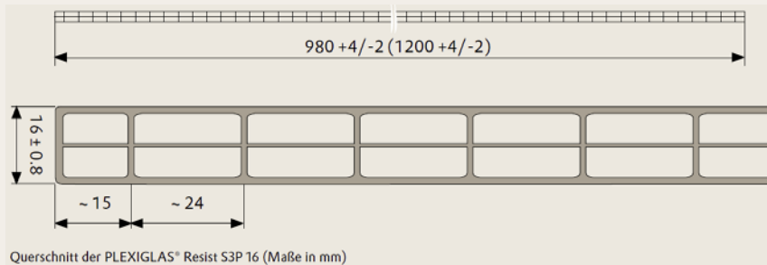
Querschnitt der PLEXIGLAS® Resist S3P 16 (Maße in mm)
