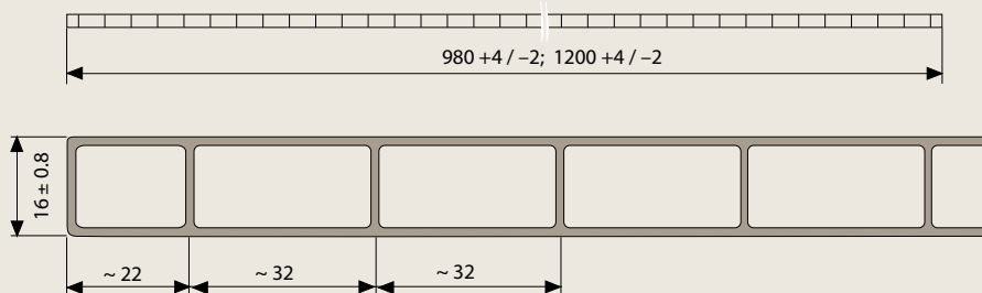
Querschnittsbild der PLEXIGLAS® Heatstop Cool Blue SDP 16 (Maße in mm)
